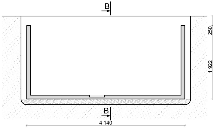
PRZEKRÓJ A-A
