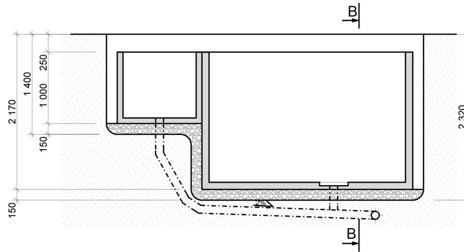
PRZEKRÓJ A-A
