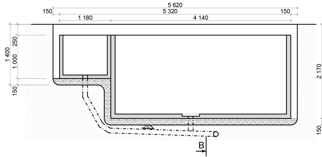
PRZEKRÓJ A-A
