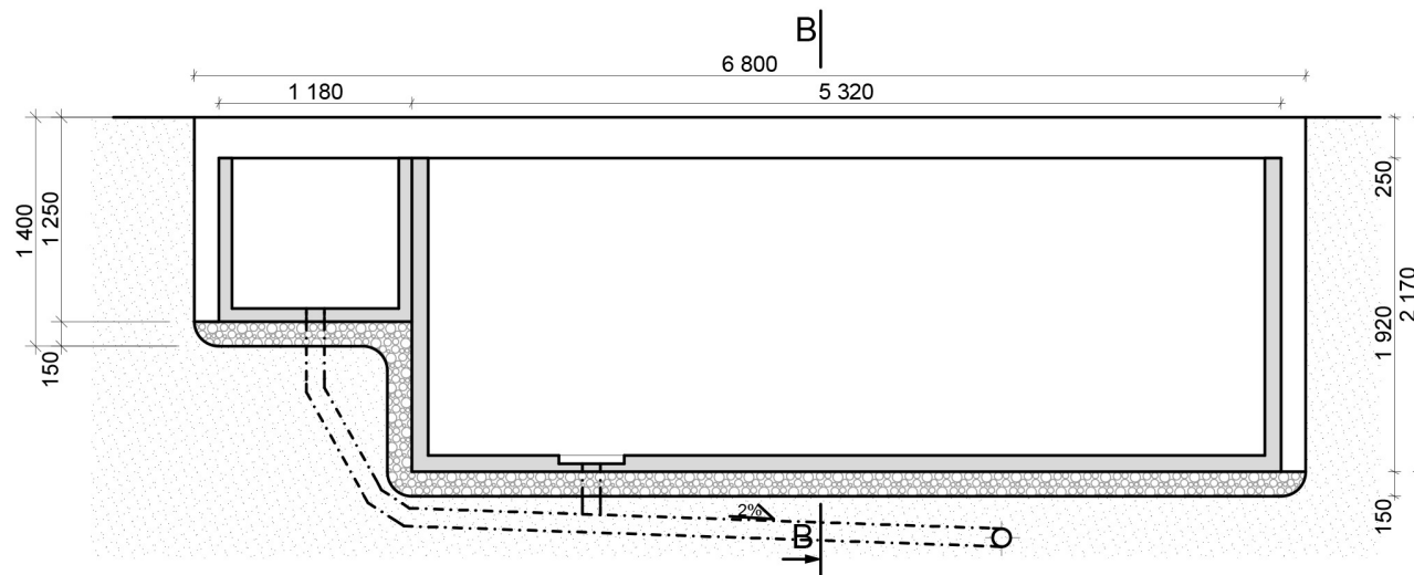
PRZEKRÓJ A-A
