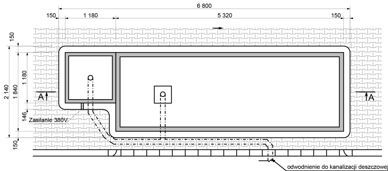
RZUT Z GÓRY
